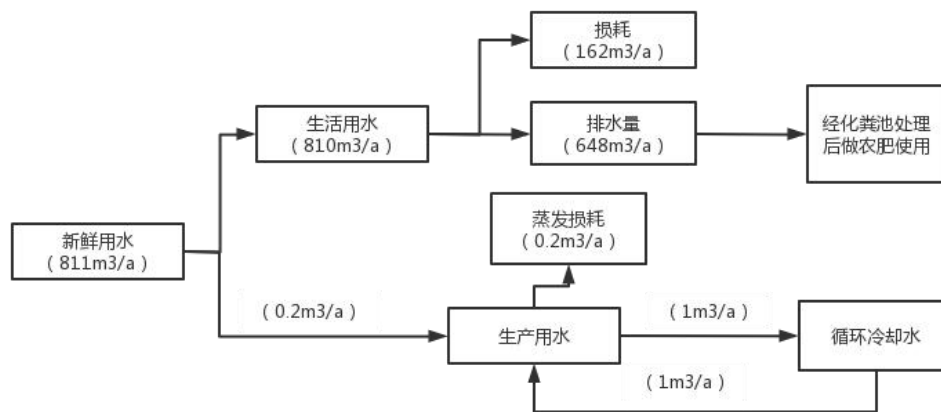
图 2-2 水平衡图
