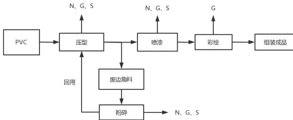
图 2-3 项目工艺流程及产污环节图
