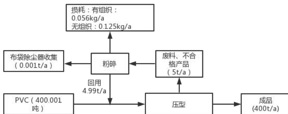
图 2-1 物料平衡图
